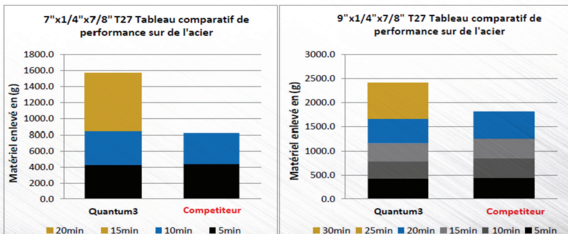
Les tableaux 2 et 3 représente la performance de la meule 7 et 9 pouces. Les deux meules ont été utilisées au maximum.
